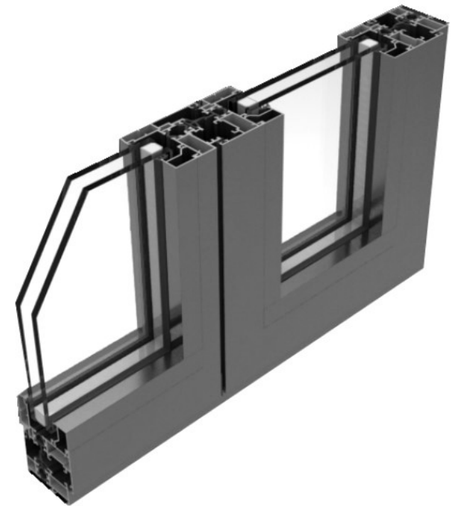
Sección abatible
