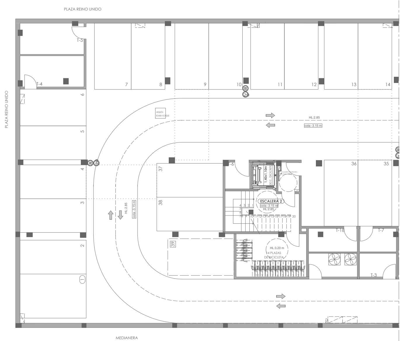
Planta Sótano -1 Escalera 2 ESCALA 1:150
